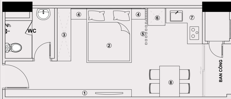
MẶT BẰNG BỐ TRÍ NỘI THẤT CĂN HỘ CH-STUDIO
